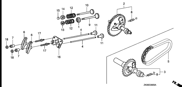
CAMSHAFT
